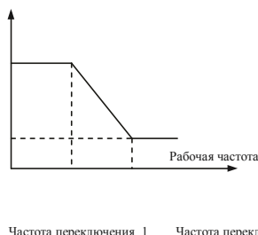
Частота переключения 1 Частота переключения 2
