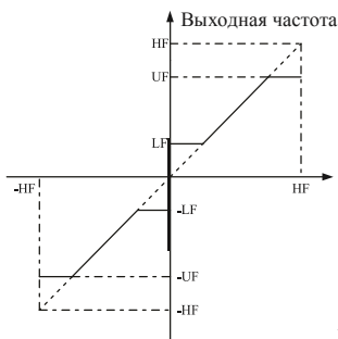
Команда выбора частоты
