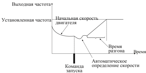
P1.0.10=1 Пуск с отслеживанием скорости
