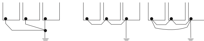
(a) Правильно (b) Неправильно (c) Не рекомендуется
