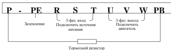
Схема подключения сети питания Модели 3 серии MCI
