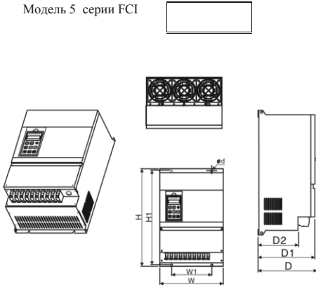
Модель 5 серии FCI
