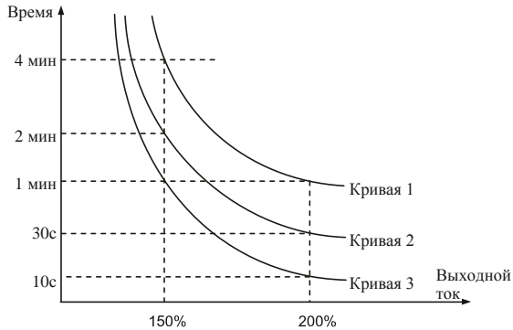
Обратнозависимые кривые перегрузки
