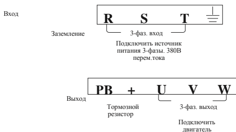
Схема подключения сети питания Модели 1, 2 серии MCI
